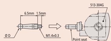
Końcówki do modeli uniwersalnych 513-304GE, 513-304GT
