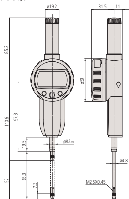
Modele o zakresie 50,8 mm
